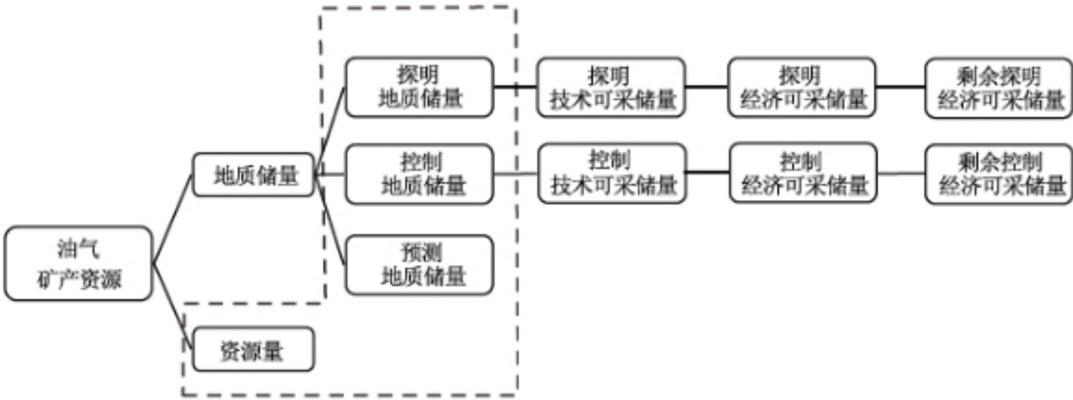
图 A.1 油气矿产资源储量类型及估算流程图 (引自 GB/T 19492)
